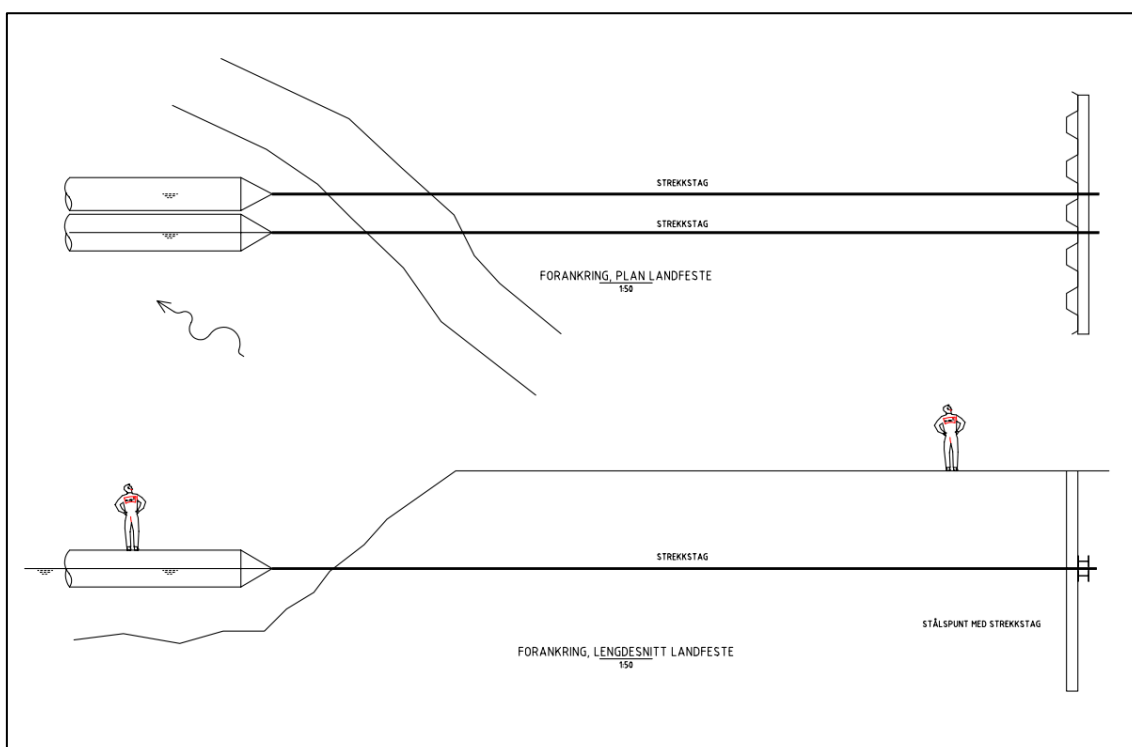
Figur 9. Lensene i fellekonstruksjonene foreslås forankret i elvebreddene på begge sider med stålpunt med strekkstag. Figuren er utarbeidet av Sweco.
