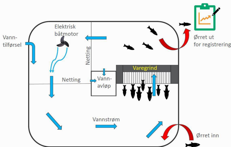
Figur 2. Skisse av settfiskkummen med innretninger for å gjøre forsøk med ulike lysåpninger i varegrinda og varierende vannhastigheter. Figuren er utarbeidet av Multiconsult.
