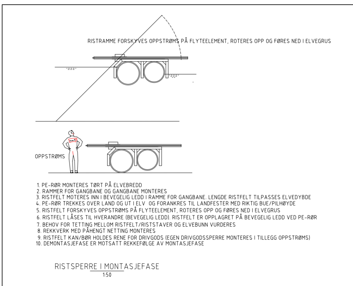
Figur 8. For å forenkle montering og demontering av fellekonstruksjoner i store elver, bør mest mulig av arbeidet gjøres på land. Ekspertgruppa foreslår en trinnvis montering av PE-rør, gangbane, rekkverk og ristfelt, som gjennomføres i omvendt rekkefølge når fellekonstruksjonen skal demonteres etter bruk. Figuren er utarbeidet av Sweco.
