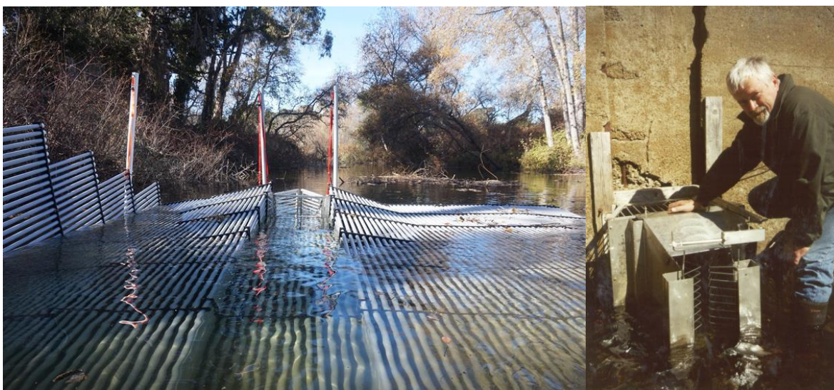
Bildeserie 4. For å sikre at større individer av nedvandrende fisk kan passere fellekonstruksjoner, er det nødvendig å lage en eller annen form for nedvandringsløsning. I Carmel River i California er det laget en nedvandringsslusning for regnbueaure i en flyteristfelle (venstre bilde). For å hindre at fisk svømmer opp gjennom nedvandringsslusningen, kan det benyttes en sluse med et fjærbelastet system som i Myhre-telleren (høyre bilde). Carmel River: www.fishbio.com . Myhre-teller: Gunnbjørn Bremset, NINA.
